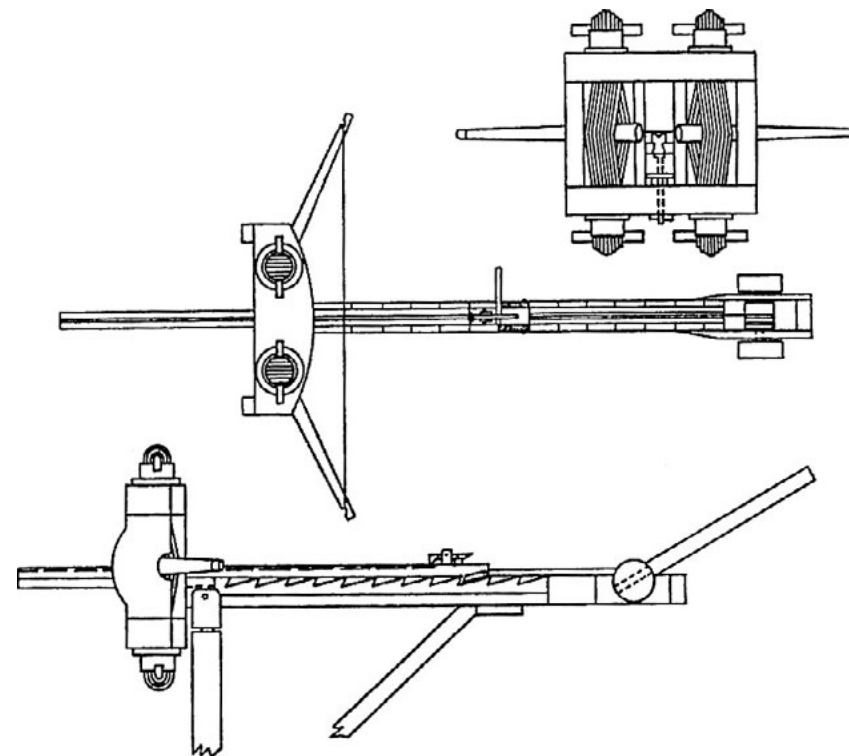
7. kép: Torziós szerkezetű nyílvetőgép (MARSDEN 1969, 34.).
