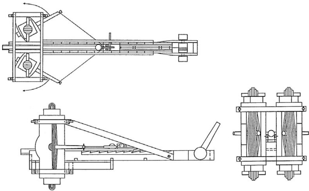
8. kép: Torziós szerkezetű kőhajítógép (MARSDEN 1969, 34.).
